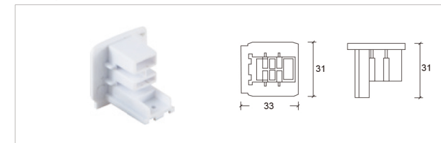
End cap
